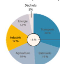
Emissions et absorption de GES en France en 2017 (source : Citepa)
