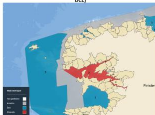
Etat chimique des masses d'eau en 2017 (source : Atlas Ifremer DCE)
